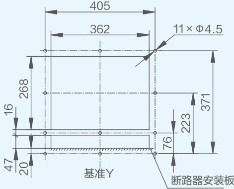
面板
