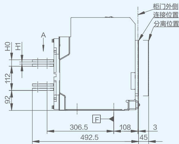
侧视图
