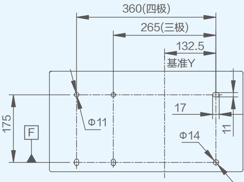
开孔尺寸 底座
