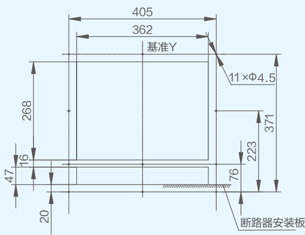
面板
