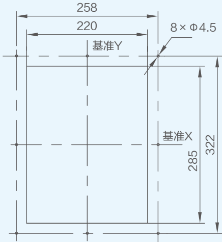
面板
