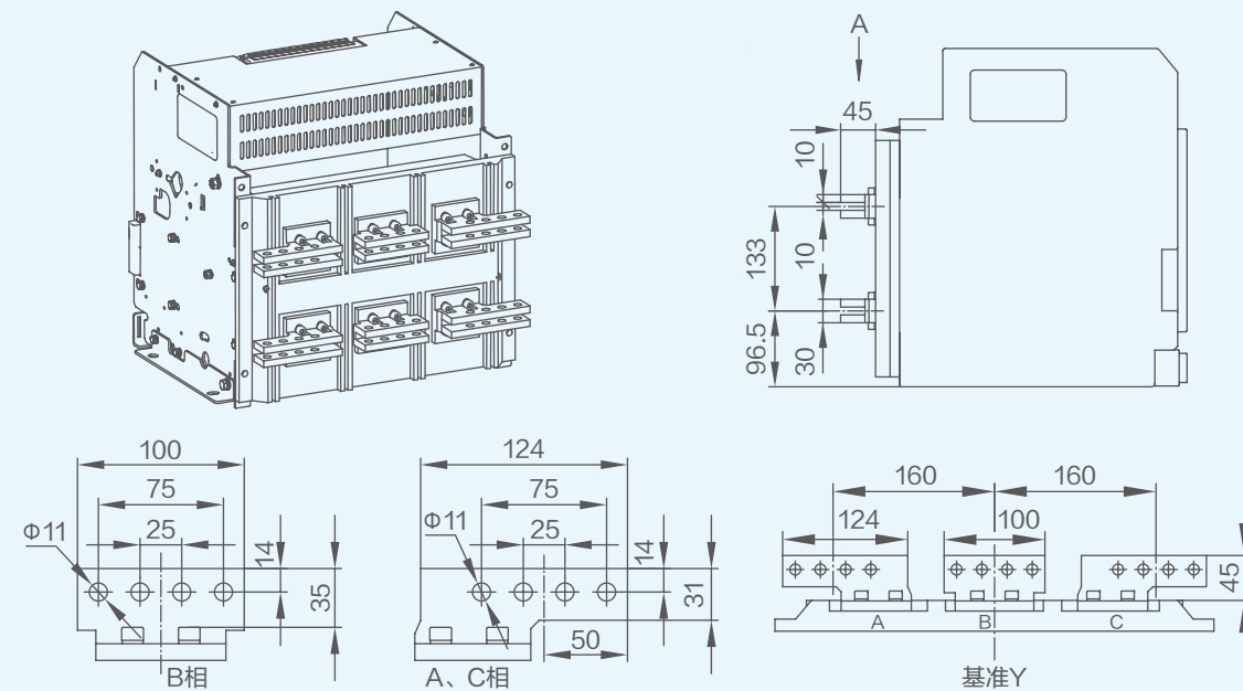
水平连接 (默认) In=3200A~4000A/3P
