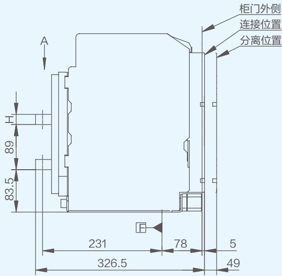
侧视图
