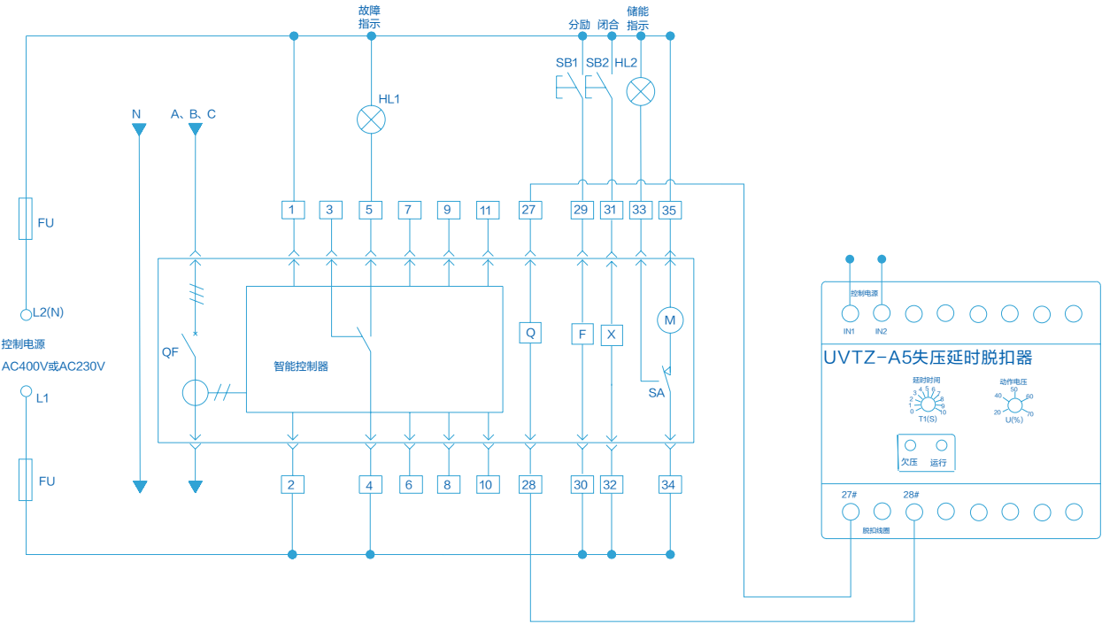
UVTZ 失压延时脱扣器接线图
