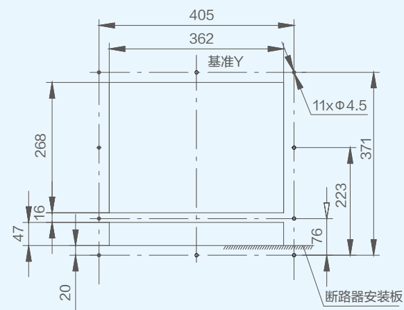
面板
