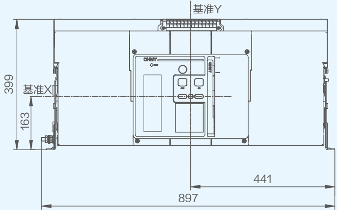
NA5-6300 固定式 正视图
