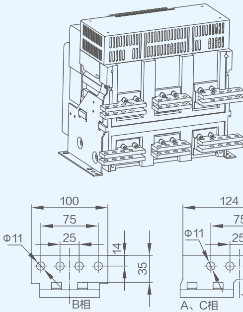
水平连接 (默认) In=3200A~4000A/3P
