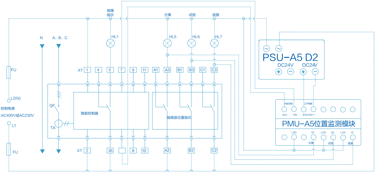
PMU 位置监测模块接线图
