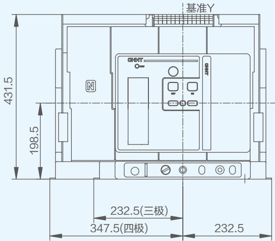
NA5-4000 抽屉式 正视图
