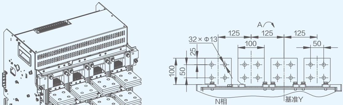
接线图 水平连接 (默认)
