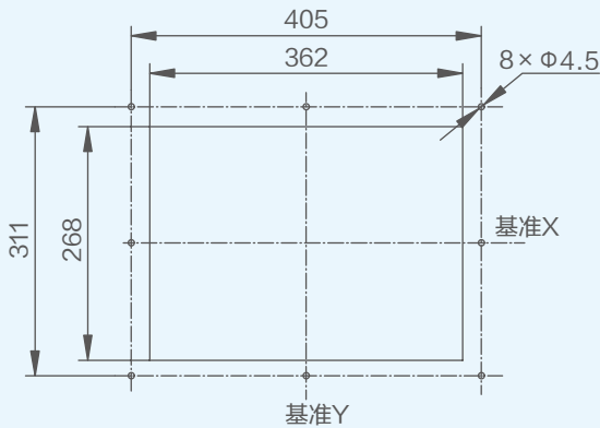
面板
