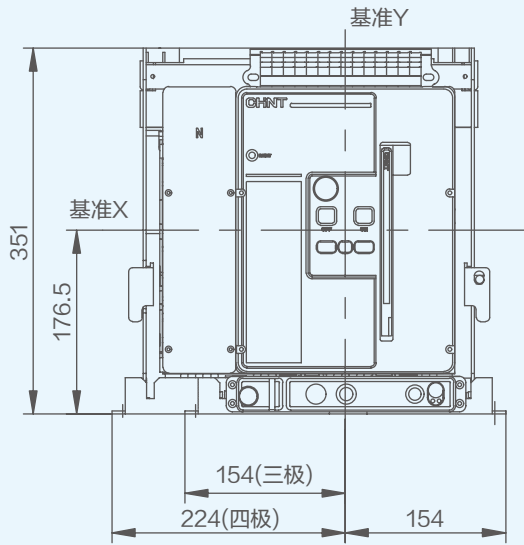
NA5-1600 抽屉式 正视图
