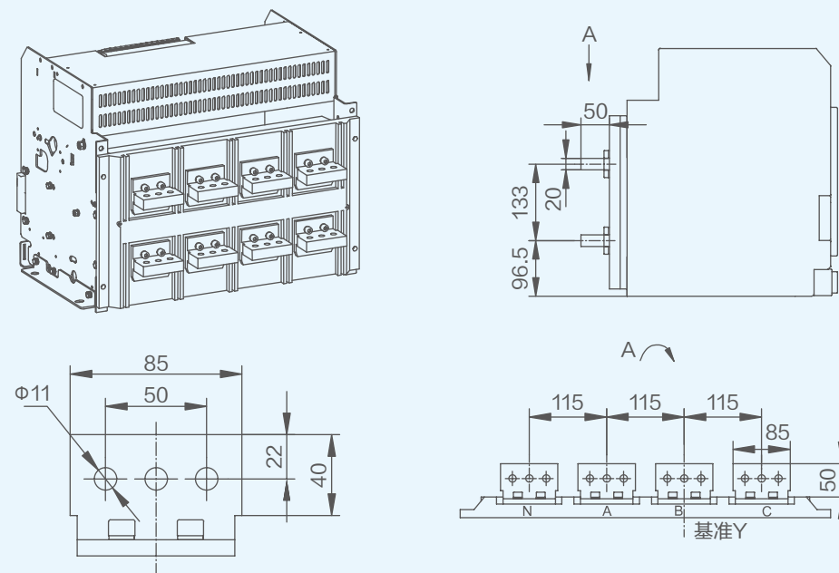
接线图 水平连接 (默认) In=800A~2500A
