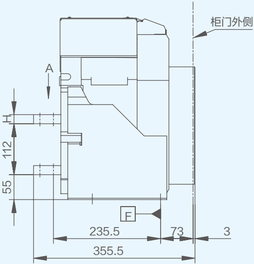
侧视图
