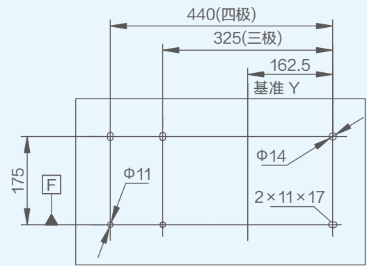
开孔尺寸 底座
