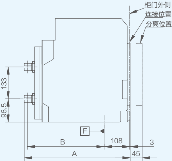
侧视图
