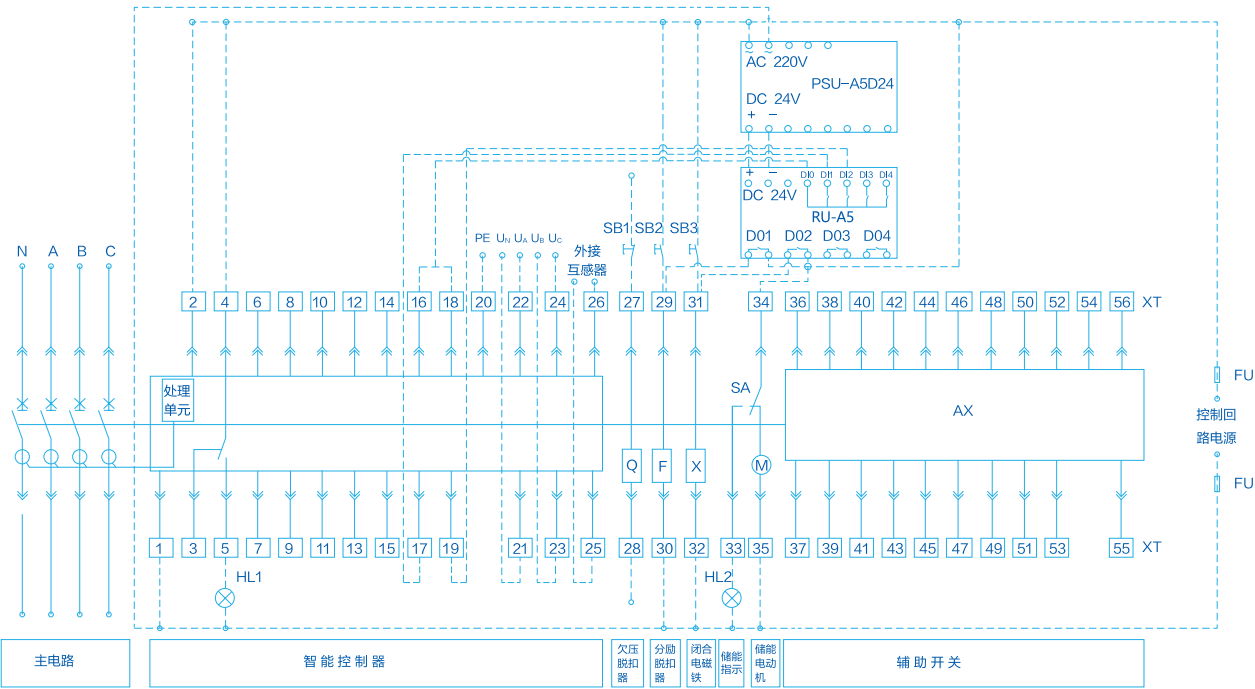
AX 辅助触头型式
