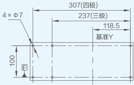
开孔尺寸 底座
