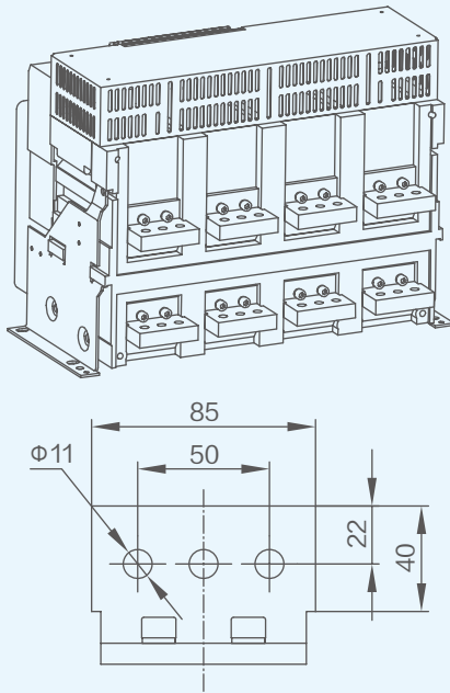
接线图 水平连接 (默认) In=800A~2500A
