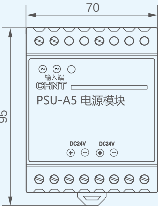
PSU 电源模块 PSU-A52 D2
