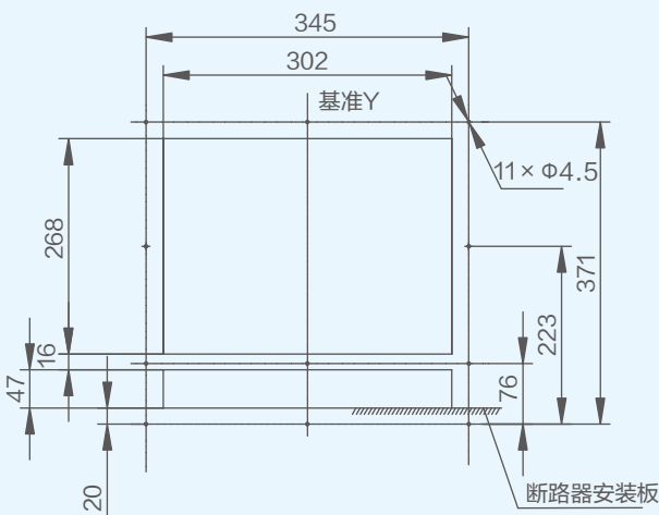
面板
