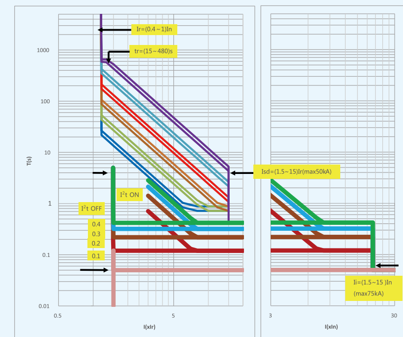
过电流保护特性曲线 I 4 T
