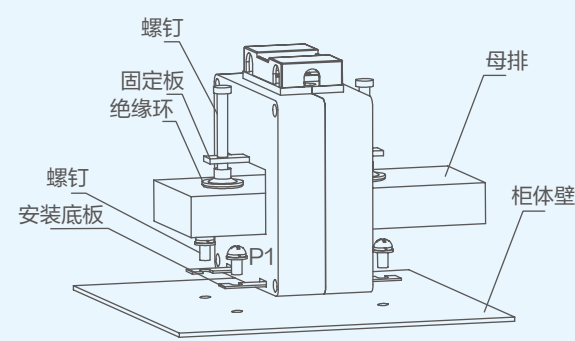
安装示意图
