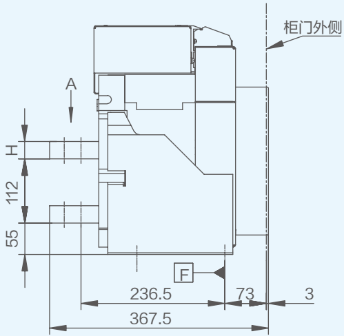
侧视图
