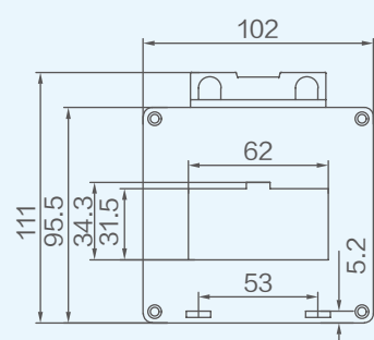
CTN-A5H10 互感器
