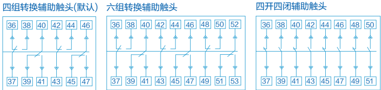
AX 辅助触头型式
