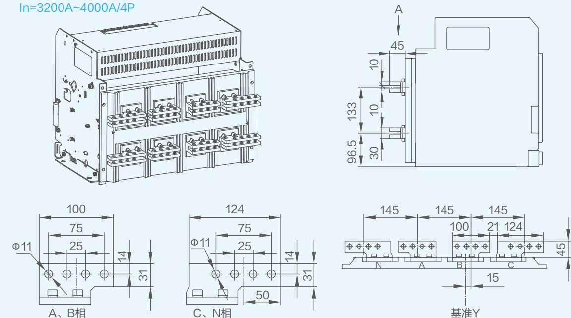
接线图 水平连接 (默认) In=3200A~4000A/4P
