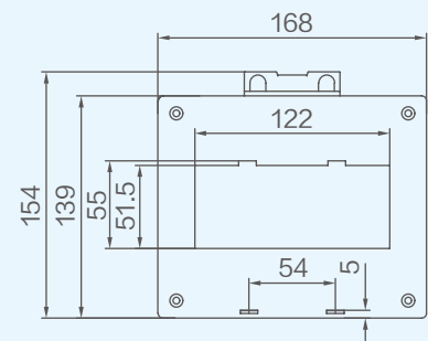
正视图
