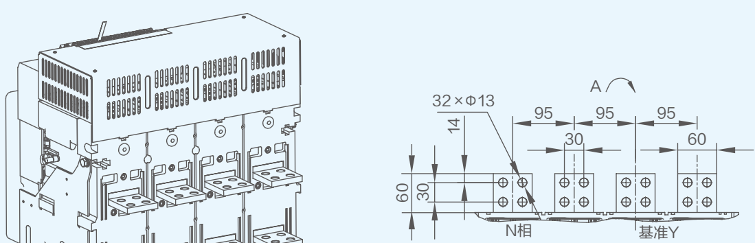
接线图 水平连接 (默认)
