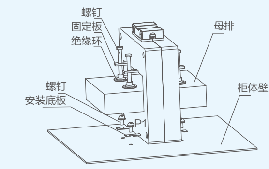
安装示意图
