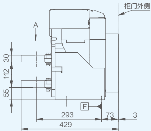
侧视图
