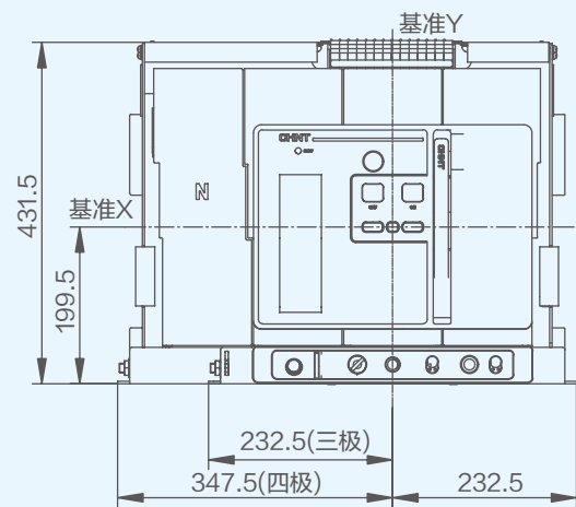
NA5-3200 抽屉式 正视图
