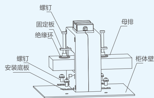
安装示意图
