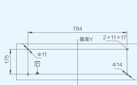
开孔尺寸 底座
