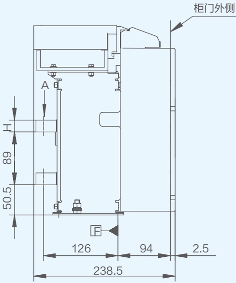
侧视图
