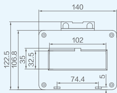
CTN-A5H12 互感器
