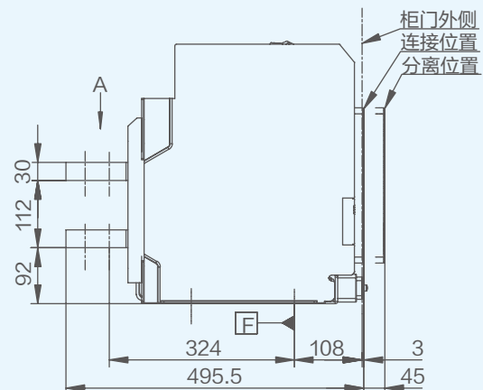
侧视图
